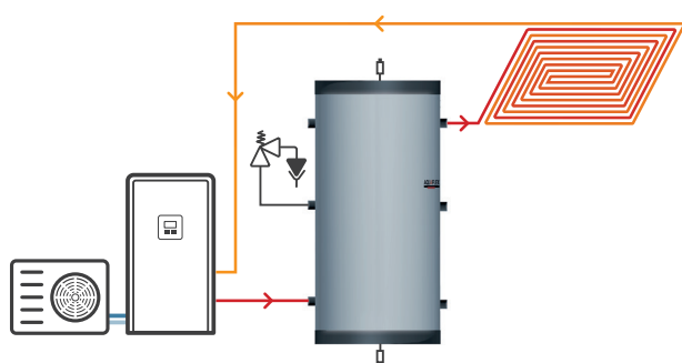
Instalación 2 tubos
